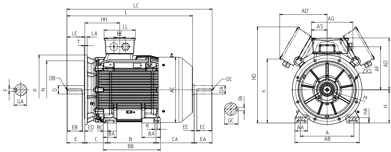
IM B35 安装方式 Type of construction IM B35
