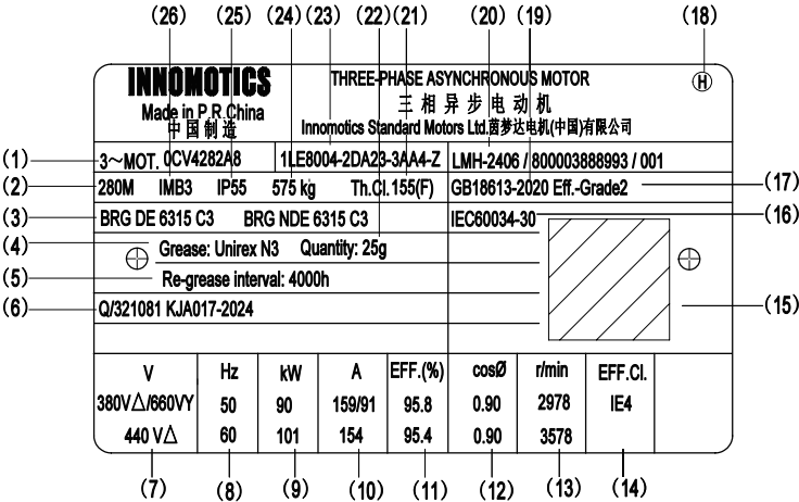
1LE8004 铸铁系列电机铭牌 1LE8004 Cast iron motor nameplate
