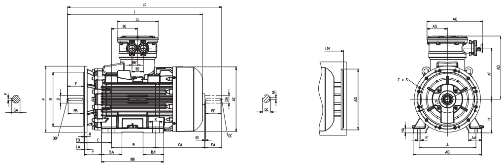
IM B35 安装结构型式 Type of construction IM B35
